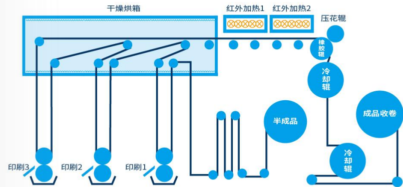
印刷、压纹线流程图-三版印刷, 压花
