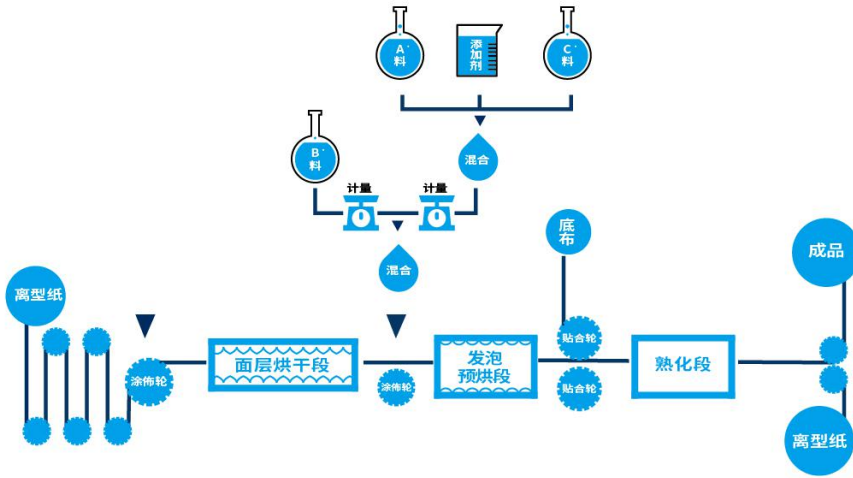
无溶剂高速混合配料加工流程图
